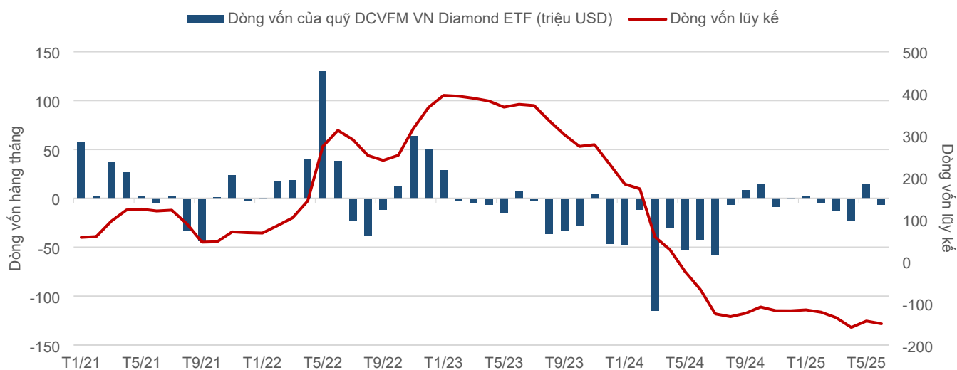
Biểu đồ 5: Dòng vốn theo tháng của quỹ DCVFM VN Diamond ETF (triệu USD)
